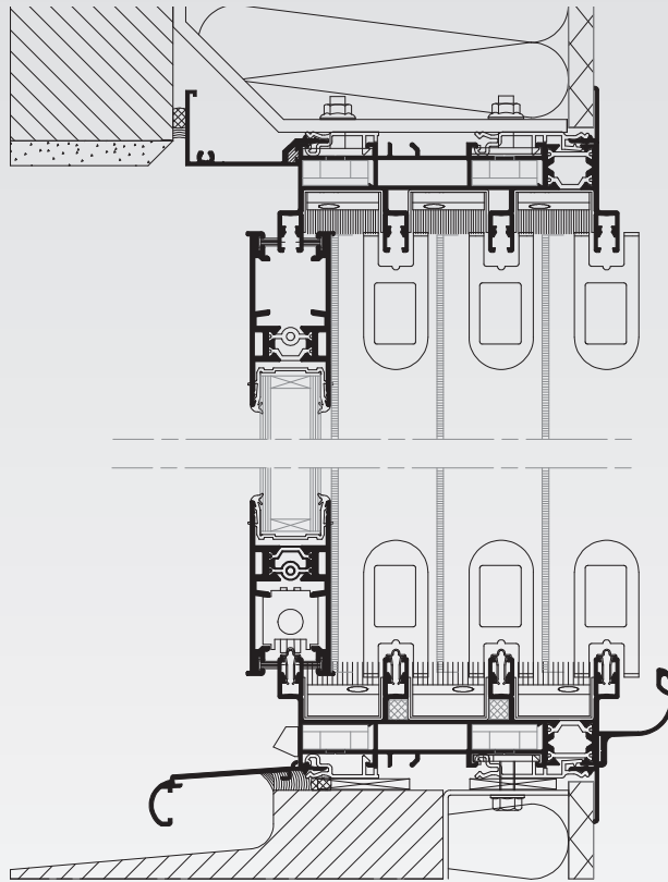
COUPE VERTICALE
