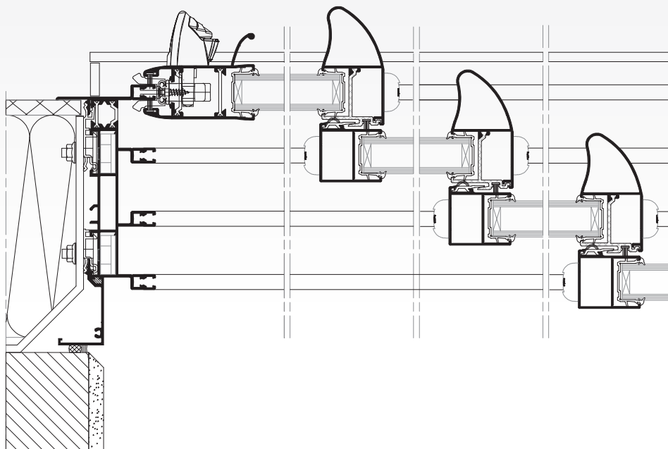
COUPE HORIZONTALE
